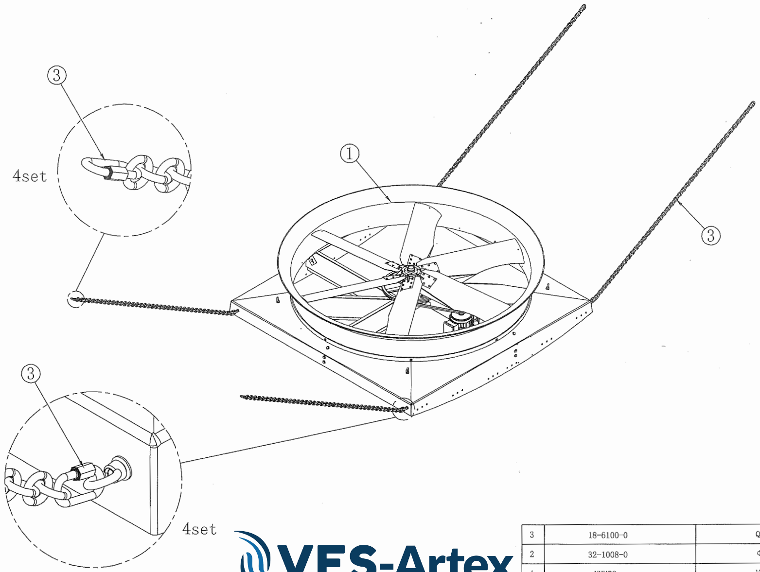
PIG-019-ECVC72_Chain_Install
